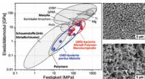
Im Elektronenmikroskop kann man die Netzwerkstruktur des porösen Titans erkennen. Das mit Polymer infiltrierte Material belegt einen bis dato unbesetzten Platz in der Karte mechanischer Eigenschaften für Strukturwerkstoffe. Bild: HZG
