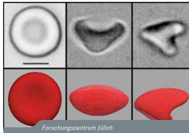
Mikroskopische Aufnahmen (oben) und Ergebnisse von Simulationen (unten) roter Blutkörperchen in Scherung. Bild: Forschungszentrum Jülich
