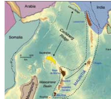
Die schwarz gestrichelte Linie zeigt, wo Bruchstücke des versunkenen Kontinents Mauritia in der Erdkruste vermutet werden. Quelle: Nature Communications; doi:10.1038/ncomms14086 (CC BY)
