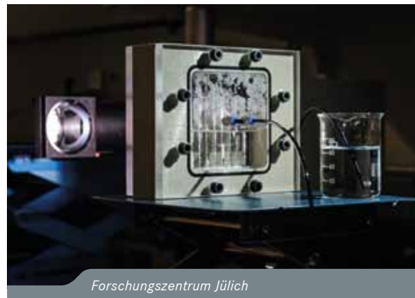
Testaufbau des Prototyps der photoelektrochemischen Wasserspaltung. Bild: Forschungszentrum Jülich/Tobias Dyck
