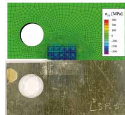
Druckeigenspannungen (bläulicher Bereich, Mitte) können Risse aufhalten. Oben: Simulation der Eigenspannungsverteilung; Unten: Laborprobe aus Flugzeug-Aluminiumlegierung mit Riss (von links kommend); Mitte: mit Laser Shock Peening behandelter Bereich. Bild: HZG
