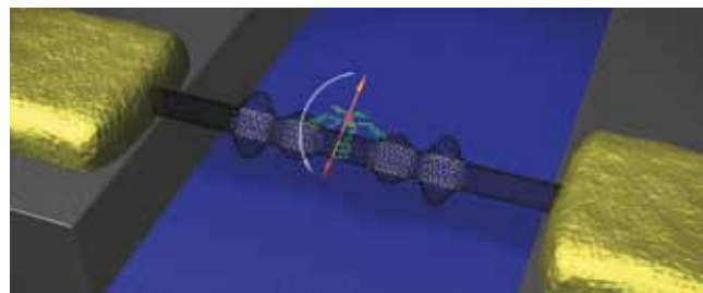
Die mechanischen Eigenschaften der Kohlenstoffnanoröhre (schwarz) bestimmen das Umklappen des Spins (orange) eines Moleküls (grün und rot). Bild: Christian Grupe/KIT
