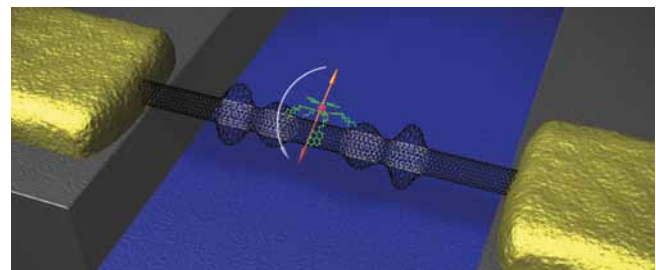
Die mechanischen Eigenschaften der Kohlenstoffnanoröhre (schwarz) bestimmen das Umklappen des Spins (orange) eines Moleküls (grün und rot). Bild: Christian Grupe/KIT
